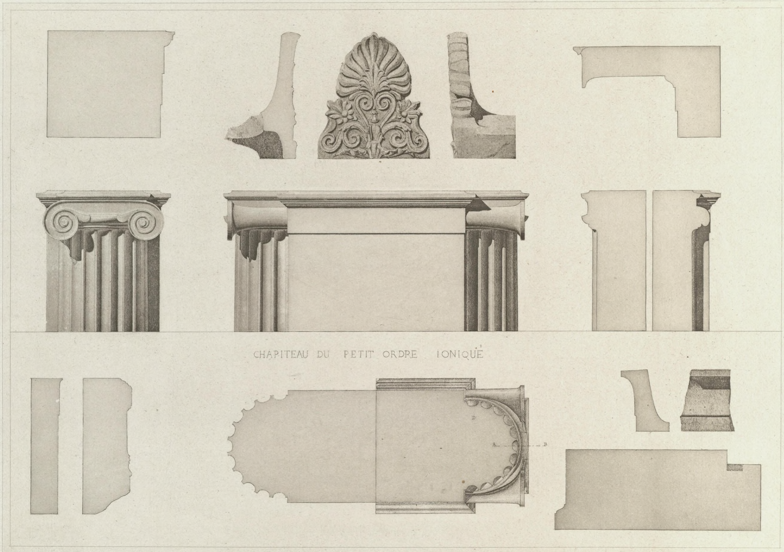
PROPYLÉE DE PALATITZA (MACÉDOINE) relevés et restauration de H. Daumet
