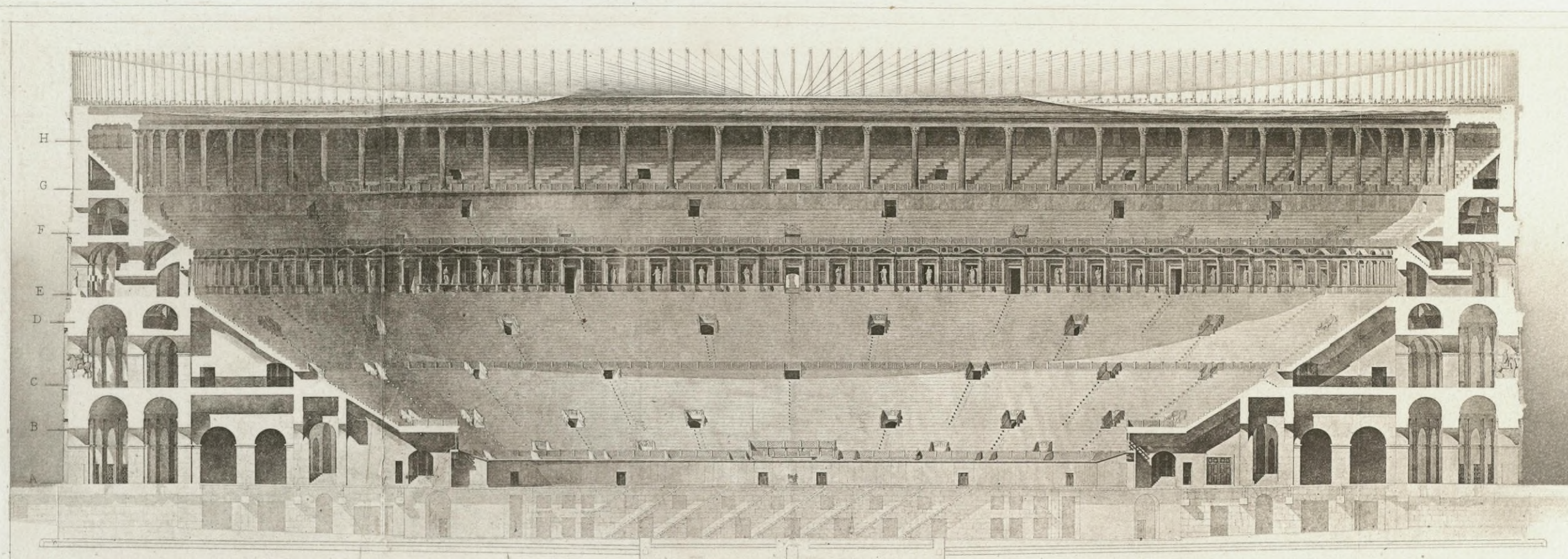
COUPE SUR LE GRAND AXE
