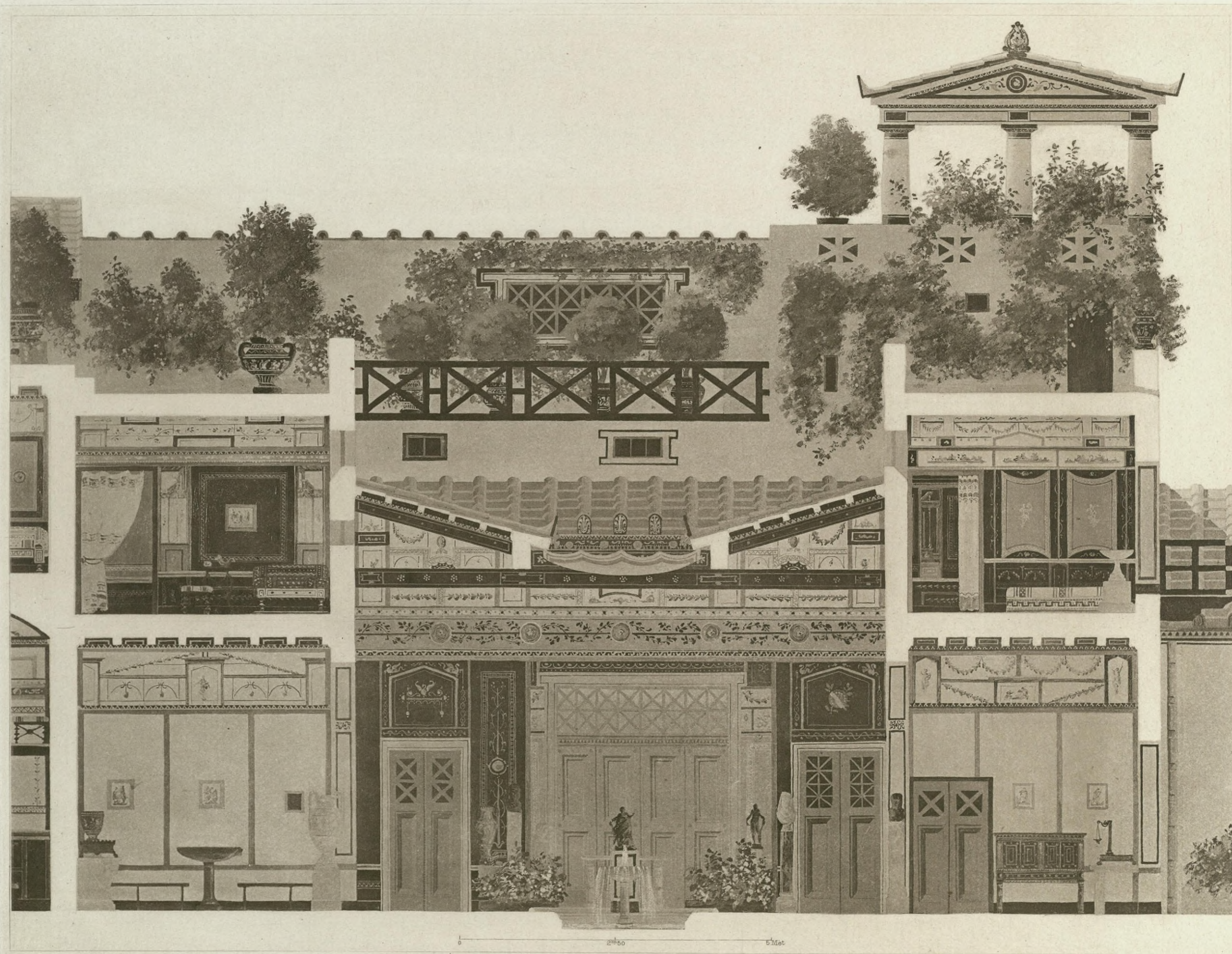
MAISON DU CENTENAIRE A POMPEÏ relevés et restauration de Chifflet 1903
