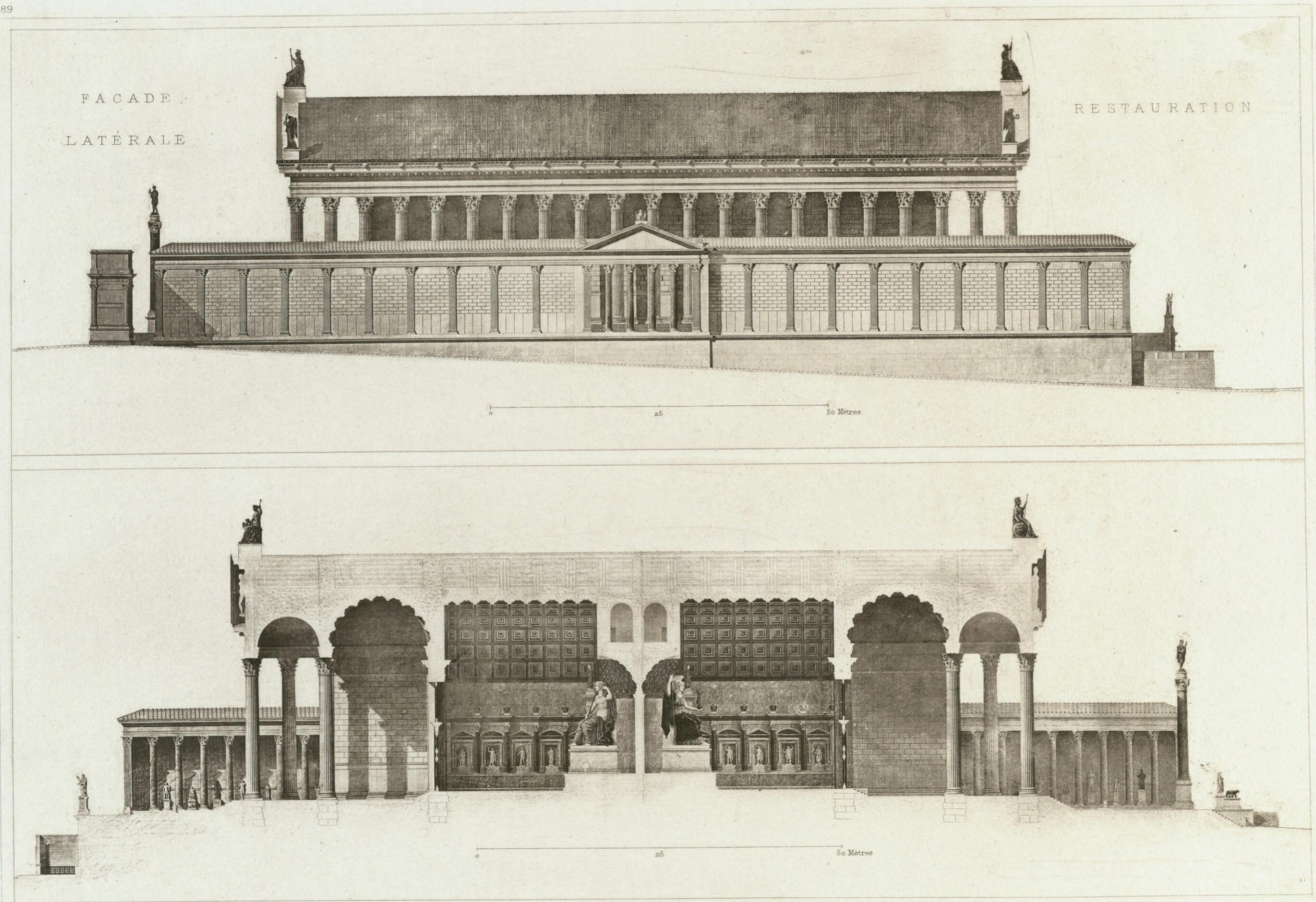
TEMPLE DE VENUS ET ROME A ROME relevés et restauration de Vaudoyer (1830)
