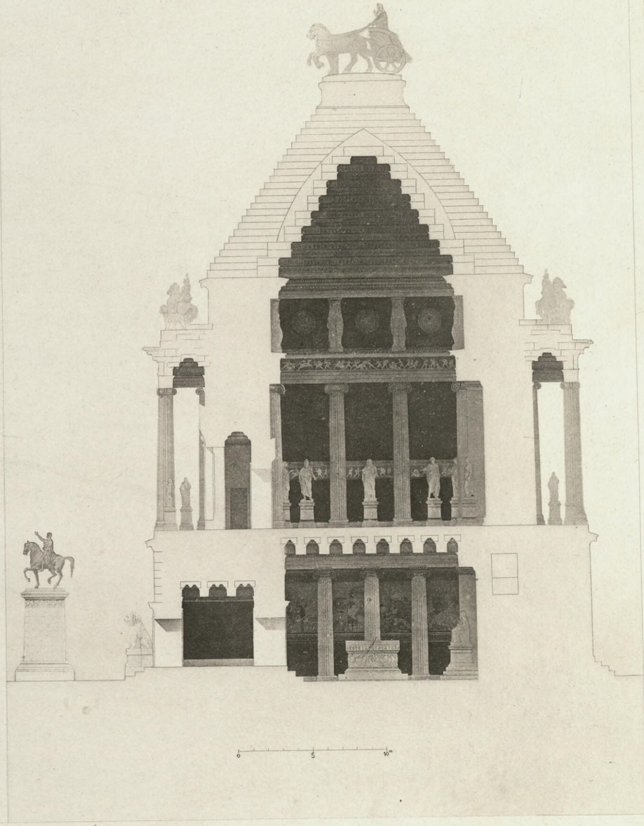
TOMBEAU DE MAUSOLE A HALICARNASSE relevés et restauration de Bernier (1877)
