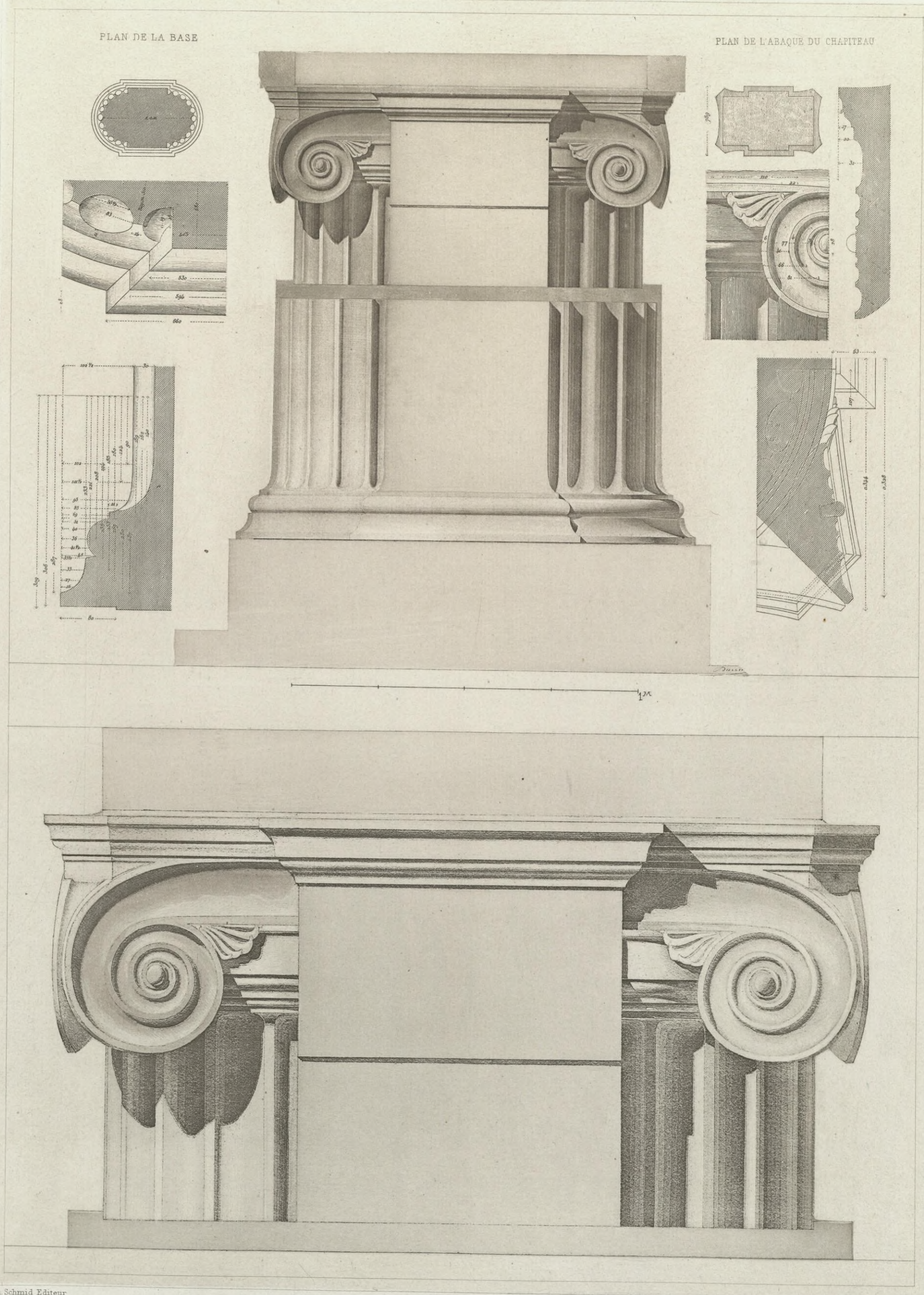
PROPYLÉE DE PALATITZA (MACÉDOINE) relevés et restauration de H. Daumet
