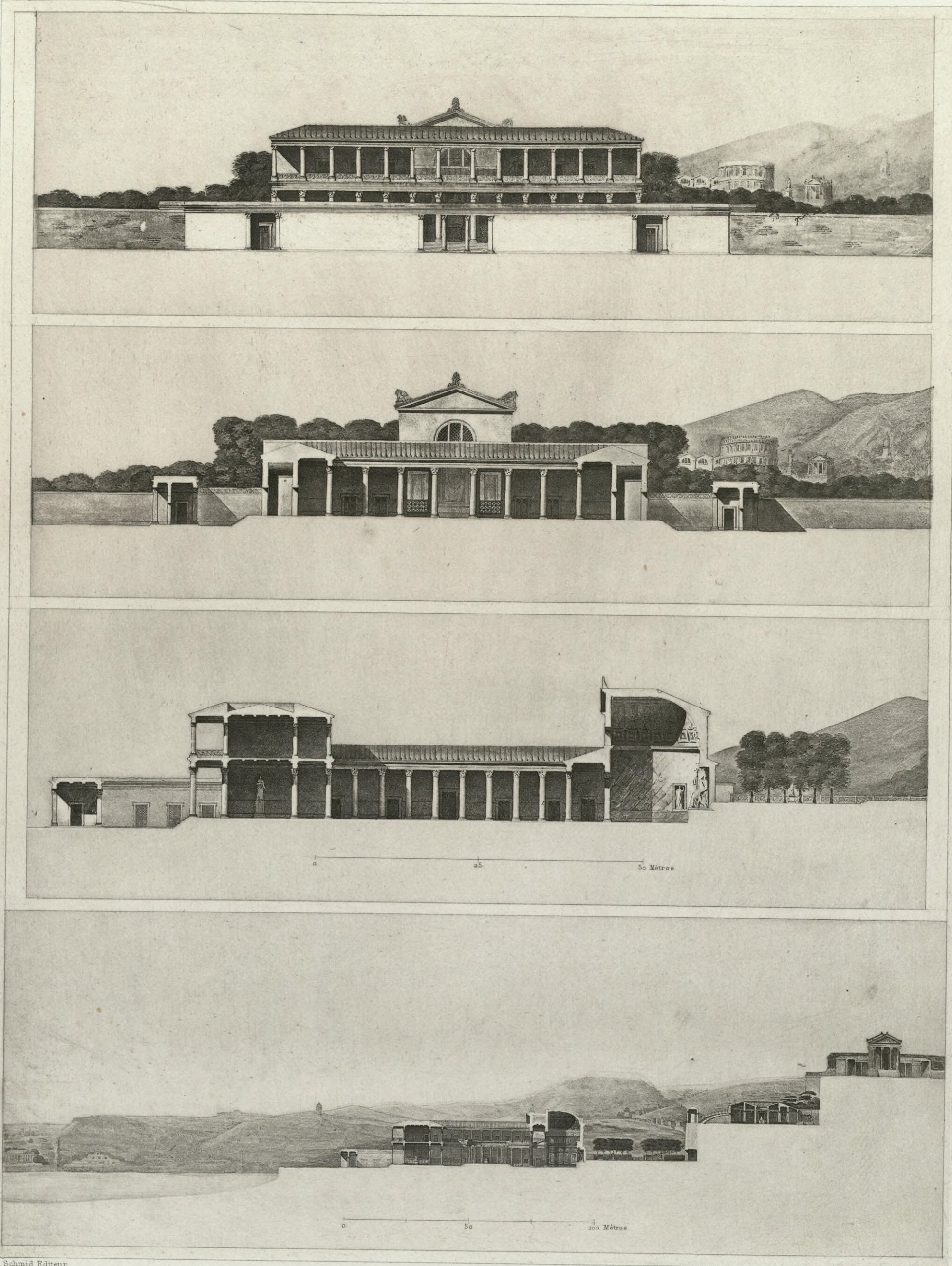
ÉDIFICE DIT TEMPLE DE SÉRAPIS A POZZOLES relevés et restauration de Caristie (1817) Voir le 1 er volume, Pl. 94
