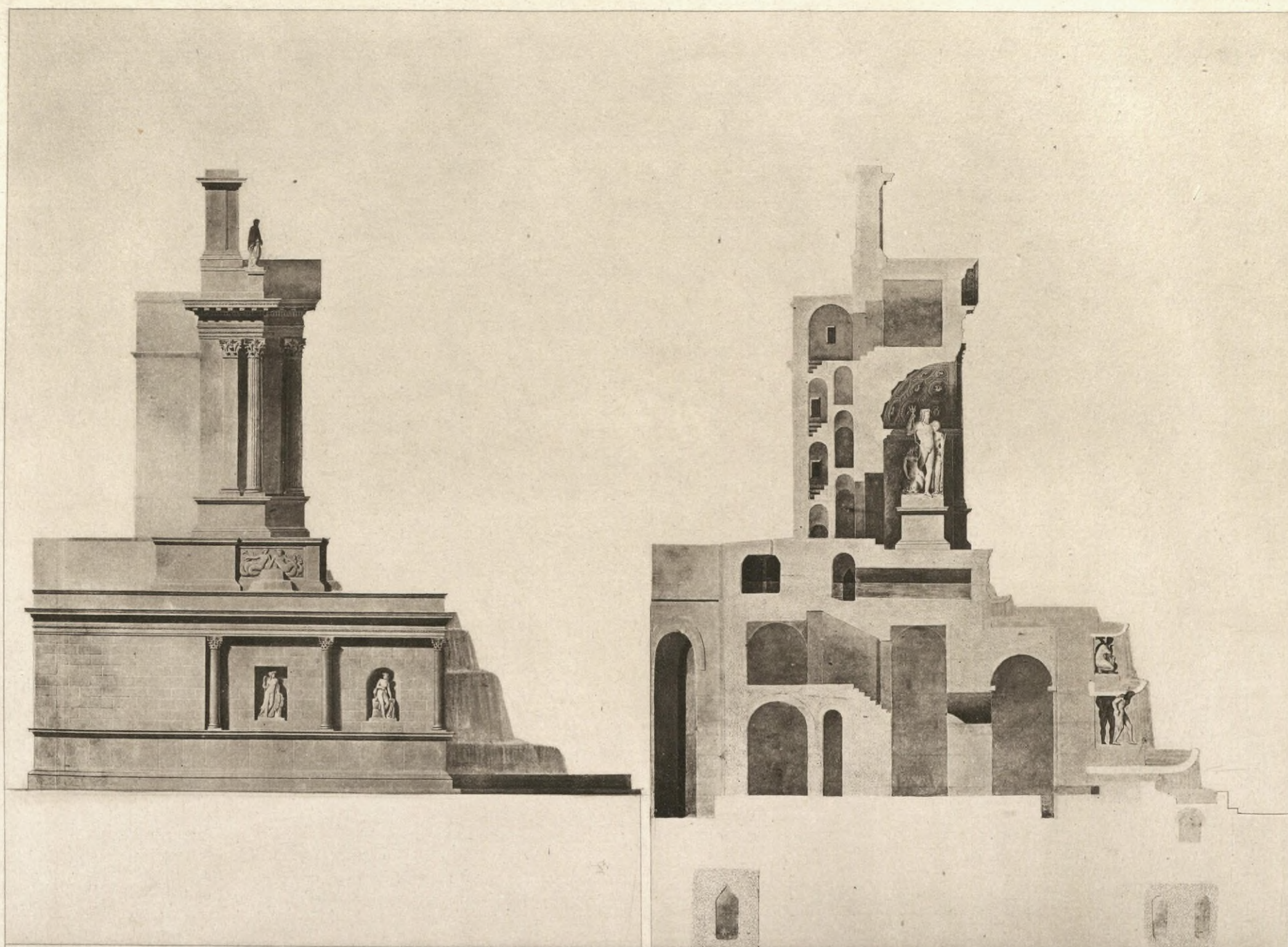
CHATEAU DE L'EAU · IVLES · FACADE · LATÉRALE · RESTAURÉE
