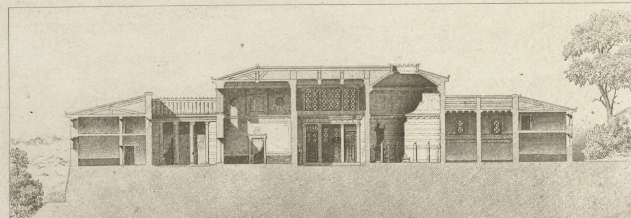
Dependances Impluvium Hestaterion Proaulion Salle du Foyer Dependances Coupe transversale sur la ligne BC
