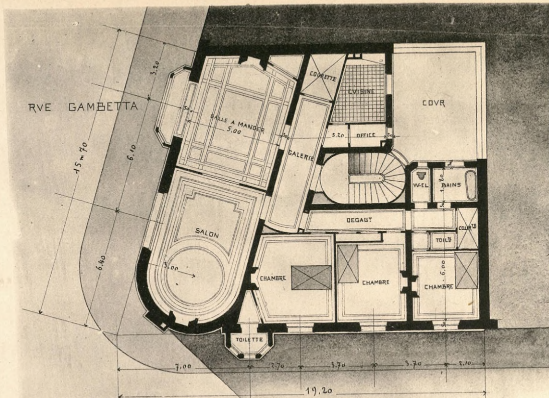
Plan du 1 er Etage
